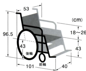
●型式:OS-12TR ●メーカー:松永製作所 ●折りたたみサイズ(cm):全幅27 ●チルト角度:0°~25° ●リクライニング角度:90°~115° ●材質:アルミ
