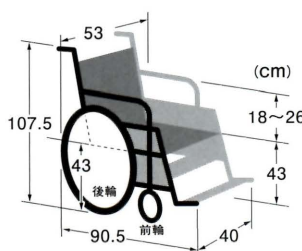
●型式:OS-12TRSP ●メーカー:松永製作所 ●折りたたみサイズ(cm):全幅27 ●チルト角度:0°~25° ●リクライニング角度:90°~115° ●材質:アルミ
